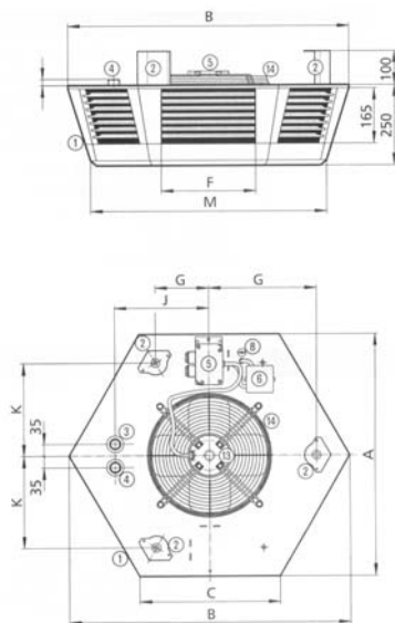
Abmessungen
