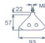
Abmessungen Querschnitt
