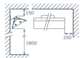
Mindestabstände Wand/Decke/Boden
