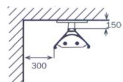
Mindestabstände Wand/Decke
