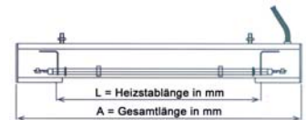
Abmessungen Seitenansicht
