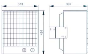
Abmessungen HAVR 3-15
