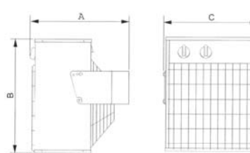
Abmessungen HSAV
