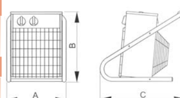
Abmessungen HPROFF 221 - 1543
