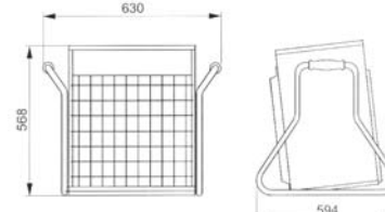
Abmessungen HPROFF 2043 u. 3043
