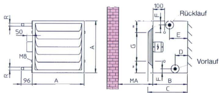
Anschlüsse in Lüftrichtung rechts
