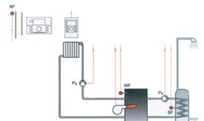
Hydraulisches Schema Smile SDC 3-10
