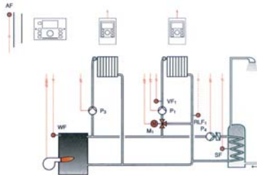
Hydraulisches Schema Smile SDC 8-10
