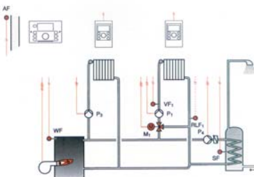
Hydraulisches Schema Smile SDC 9-21
