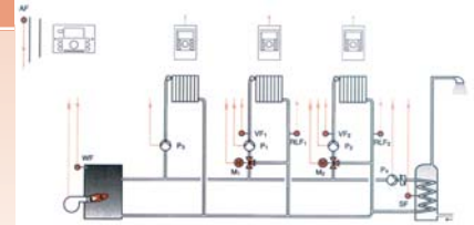
Hydraulisches Schema Smile12-31
