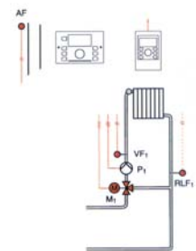
Hydraulisches Schema Smile SDC 3-40
