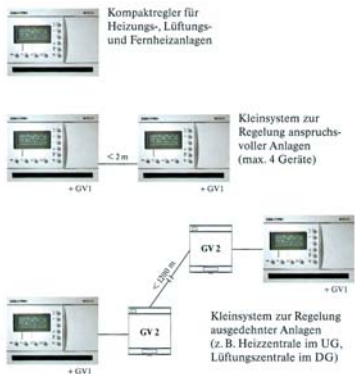
MCR 200 - Das ausbaufähige Regelsystem
