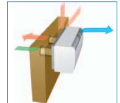
Luftfluß bei AusbläÙ nach oben im Kühlbetrieb
