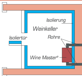
Installationsschema für C18IN
