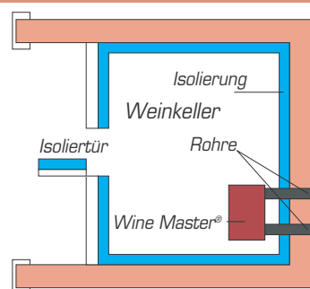
Installationsschema für C50IN
