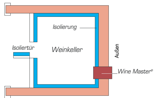
Installationsschema für C25SR und C50SR
