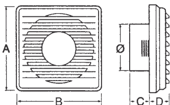
Abmessungen
