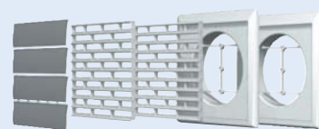
2x Gitterträger, 2x Gitter mit feststehenden Lamellen, 4x selbsthebende Lamellen
