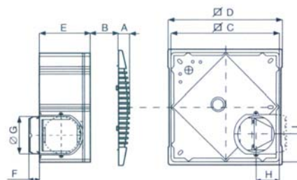
Vort Press I 140 und Vort Press I 240 (Ausblasstutzen kann für Luftrichtung nach oben oder nach hinten montiert werden)
