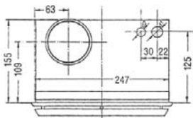
Abmessungen HGS IIK
