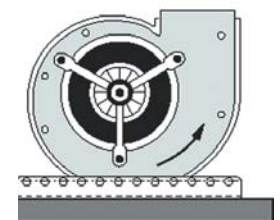
Bodenmontage
