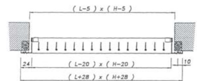
Abmessungen
