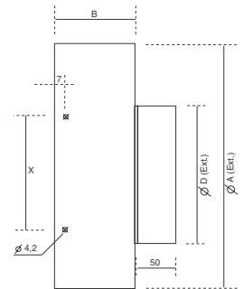
PFU 40 Abmessungen
