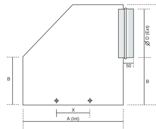
PFU 41 Abmessungen
