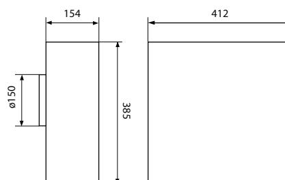
Abmessungen HAWG1100
