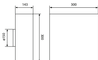
Abmessungen HAWG800
