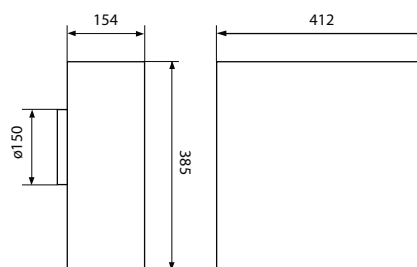
Abmessungen HAWG1100
