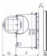
Ariett I und Vort Press 110 I mit seitlichem Ausblas (Art. Nr. 22841)
