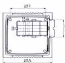
Ariett I und Vort Press 110 I mit seitlichem Ausblas (Art. Nr. 22841)
