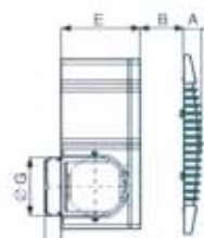
Vort Press 140 I und Vort Press 240 I (Ausblasstutzen kann für Lufrichtung rückwärtig oder seitlich nach oben montiert werden)
