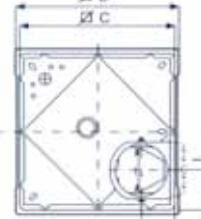
Vort Press 140 I und Vort Press 240 I (Ausblasstutzen kann für Lufrichtung rückwärtig oder seitlich nach oben montiert werden)
