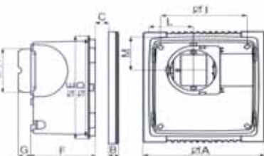
Ariett I und Vort Press 110 I mit rückwärtigem Ausblas
