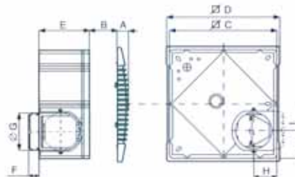
Vort Press 140 I und Vort Press 240 I (Ausblasstutzen kann für Lufrichtung rückwärtig oder seitlich nach oben montiert werden)
