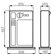
Vortronic 100
