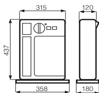
Vortronic 50
