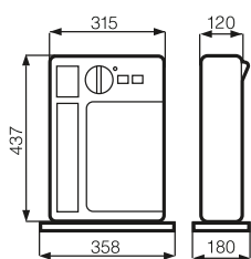
Depuro 45 H
