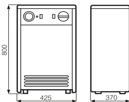
Vortronic 200 T
