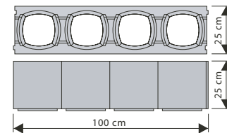
Abmessungen Poolblock Baustein
