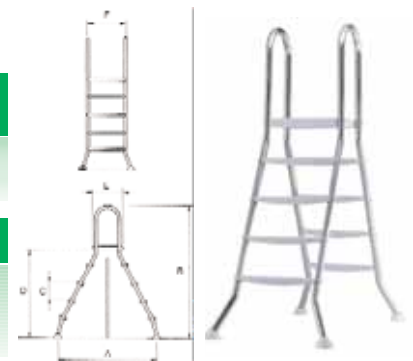
Edelstahlleiter für Aufstellbecken
